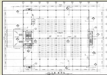
2층 평면도
